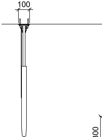
10103 PLAN
